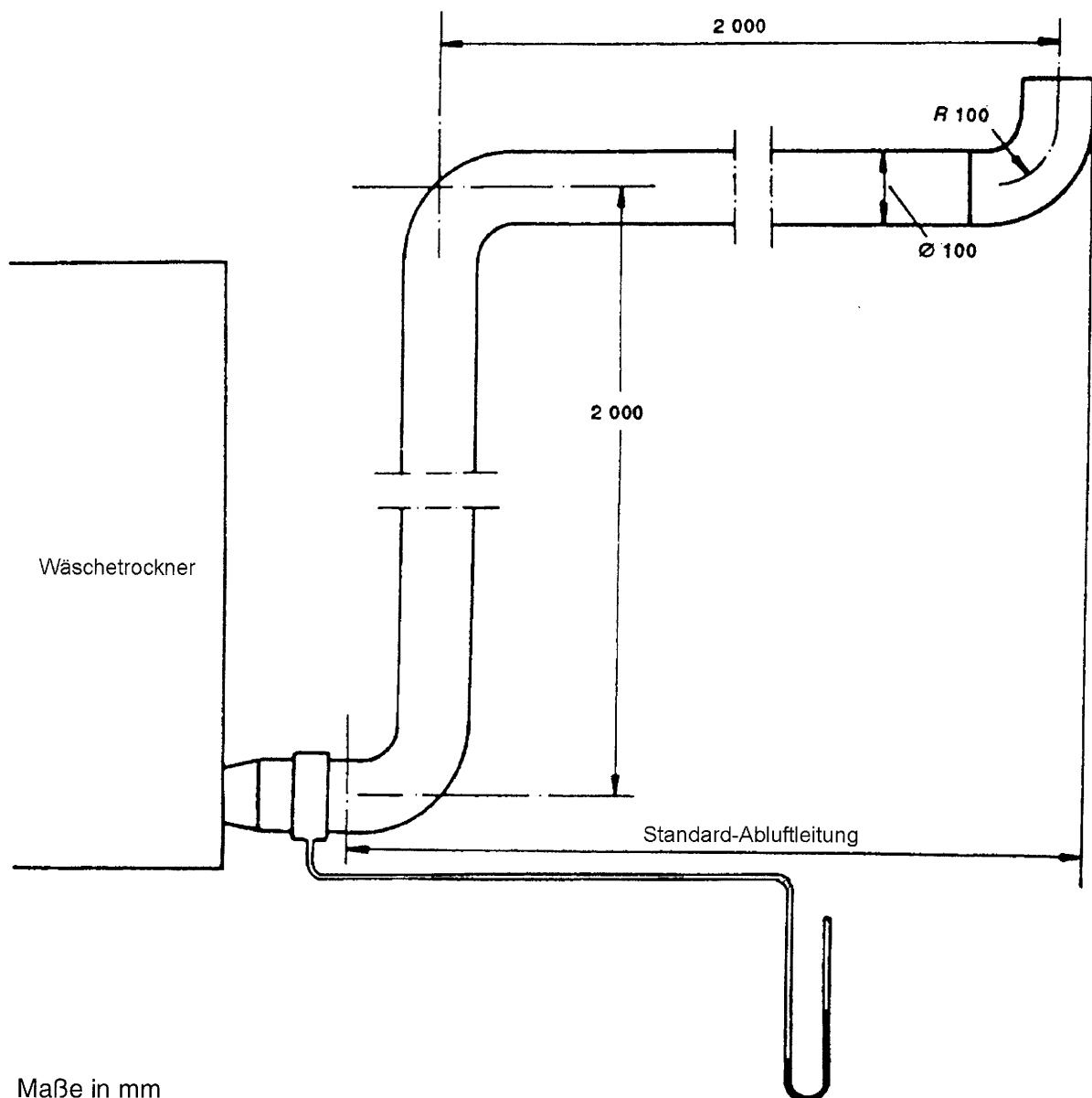
Bild A.1 – Standard-Abluftleitung
