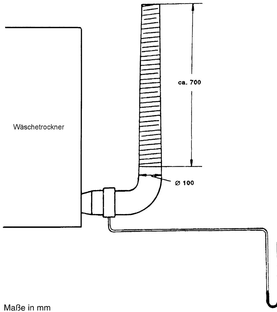
Bild A.2 – Standard-Abflutleitung-Simulator
